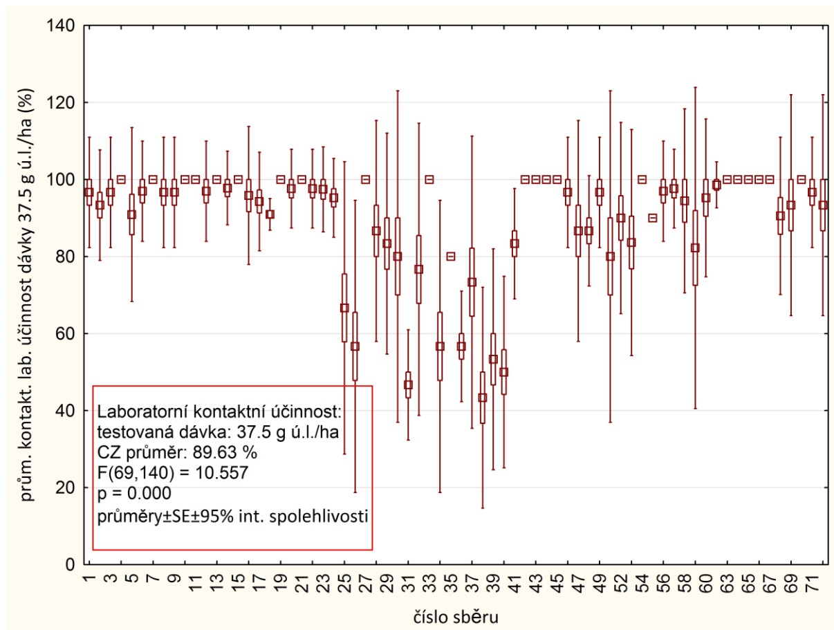
Graf 3 - Srovnání hodnot laboratorních účinností dosažených u jednotlivých populací blýskáčků 500% dávkou lambda-cyhalothrinu (= dávka 5-násobně vyšší než max. registrovaná dávka: 37,5 g.ha -1 ). Čísla populací uvedených v grafu (osa x) odpovídají číslům populací v tabulkách 3a 4 a na obr. 1. Použitá metoda testování: Adult vial test IRAC 011 version 3 (2014, 70 populací otestováno).
