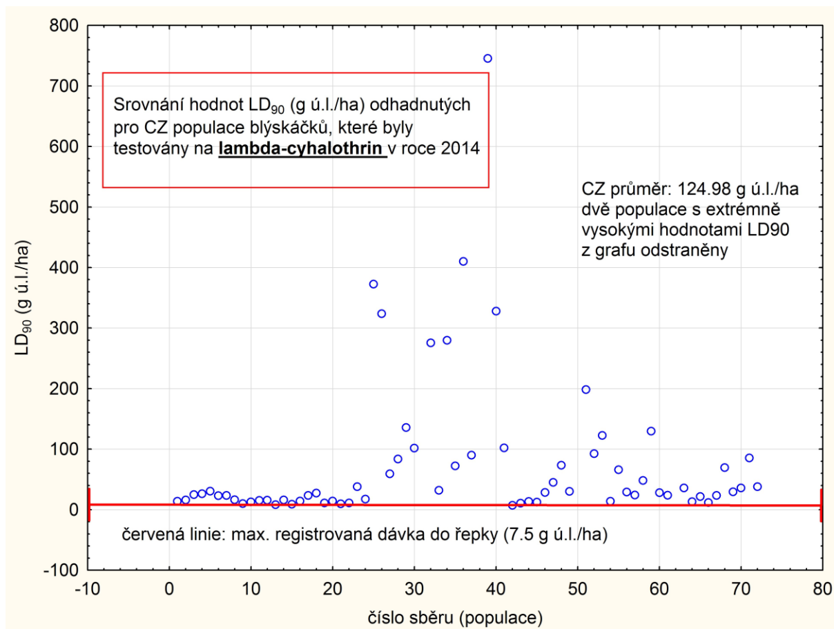
Graf 5 - Srovnání hodnot LD_{90} (g ú.l./ha) pro lambda-cyhalothrin odhadnutých (probitová regrese) pro testované populace blýskáčků v roce 2014. Červená čára vymezuje opět maximální registrovanou dávku pro lambda-cyhalothrin v řepce ozimé v ČR (7,5 g ú.l./ha). Čísla populací uvedených v grafu (osa x) odpovídají číslům populací v tabulkách 3a 4 a na obr. 1. Použitá metoda testování: Adult vial test IRAC 011 version 3 (2014, 70 populací otestováno). Poznámka : ze souboru zobrazovaném v grafu vyřazeny dvě populace (č. 31 Starovičky LD_{90} = 1600 g ú.l./ha; č. 38 Plzeň LD_{90} = 1950 g ú.l./ha) s extrémně vysokými hodnotami LD_{90} . Důvod vyloučení těchto hodnot z grafu bylo zachování sdělnosti grafu - cílem je ukázat, jaký podíl populací má hodnoty LD_{90} nad hodnotou max. registrované dávky.
