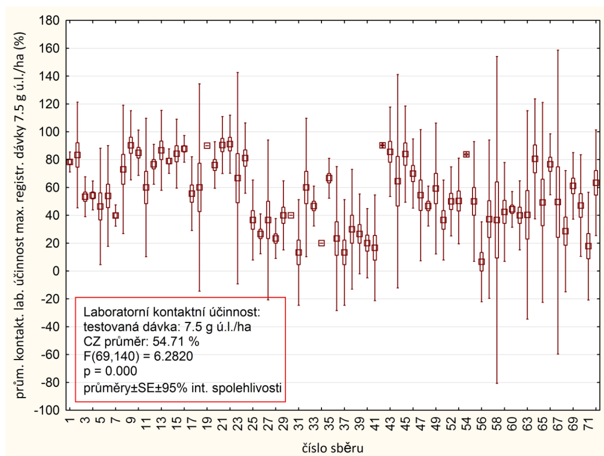
Graf 1 - Srovnání hodnot laboratorních účinnosti dosažených u jednotlivých populací blýskáčků maximální registrovanou dávkou lambda-cyhalothrinu do řepky ozimé v ČR (7,5 g.ha -1 ). Čísla populací uvedených v grafu (osa x) odpovídají číslům populací v tabulkách
