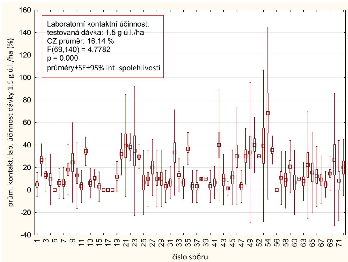
Graf 2 - Srovnání hodnot laboratorních účinností dosažených u jednotlivých populací blýskáčků 20% dávkou lambda-cyhalothrinu (= dávka 5-násobně nižší než max. registrovaná dávka: 1,5 g.ha -1 ). Čísla populací uvedených v grafu (osa x) odpovídají číslům populací v tabulkách 3a 4 a na obr. 1. Použitá metoda testování: Adult vial test IRAC 011 version 3 (2014, 70 populací otestováno).
