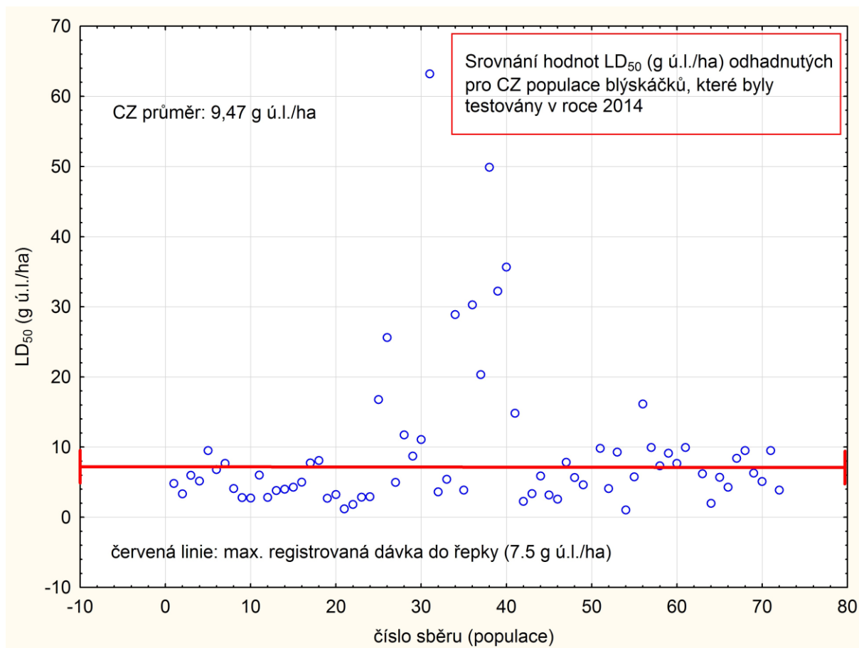
Graf 4 - Srovnání hodnot LD 50 (g ú.l./ha) pro lambda-cyhalothrin odhadnutých (probitová regrese) pro testované populace blýskáčků v roce 2014. Červená čára vymezuje maximální registrovanou dávku pro lambda-cyhalothrin v řepce ozimé v ČR (7,5 g ú.l./ha). Čísla populací uvedených v grafu (osa x) odpovídají číslům populací v tabulkách 3a 4 a na obr. 1. Použitá metoda testování: Adult vial test IRAC 011 version 3 (2014, 70 populací otestováno).
