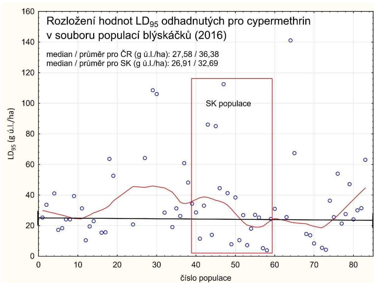
Graf 6 - Rozložení hodnot LD_{95} (g ú.l./ha) odhadnutých pro cypermethrin (probitová regrese) pro testované populace blýskáčků v roce 2016 (každé modré kolečko je jedna testovaná populace). Černá čára vymezuje registrovanou dávku pro cypermethrin v řepce ozimé v ČR (25 g ú.l./ha). Slovenské populace se v grafu nachází v červeném obdélníku. Použitá metoda testování: Adult vial test IRAC 011 version 3 (2016, 66 populací otestováno celkem; 45 z ČR + 21 z SK).
