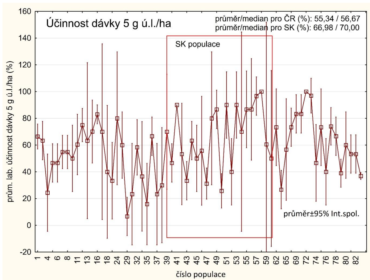
Graf 2 - Hodnoty laboratorních účinností dosažené u jednotlivých populací blýskáčků dávkou pětikrát nižší, než je dávka registrovaná (to je 5 g. ú.l./ha). Čísla populací uvedených v grafu (osa x) odpovídají číslům populací v tabulkách 4a,b a 5a,b. Použitá metoda testování: Adult vial test IRAC 011 version 3 (2016, 66 populací otestováno celkem; 45 populací z ČR, 21 populací z SK).
