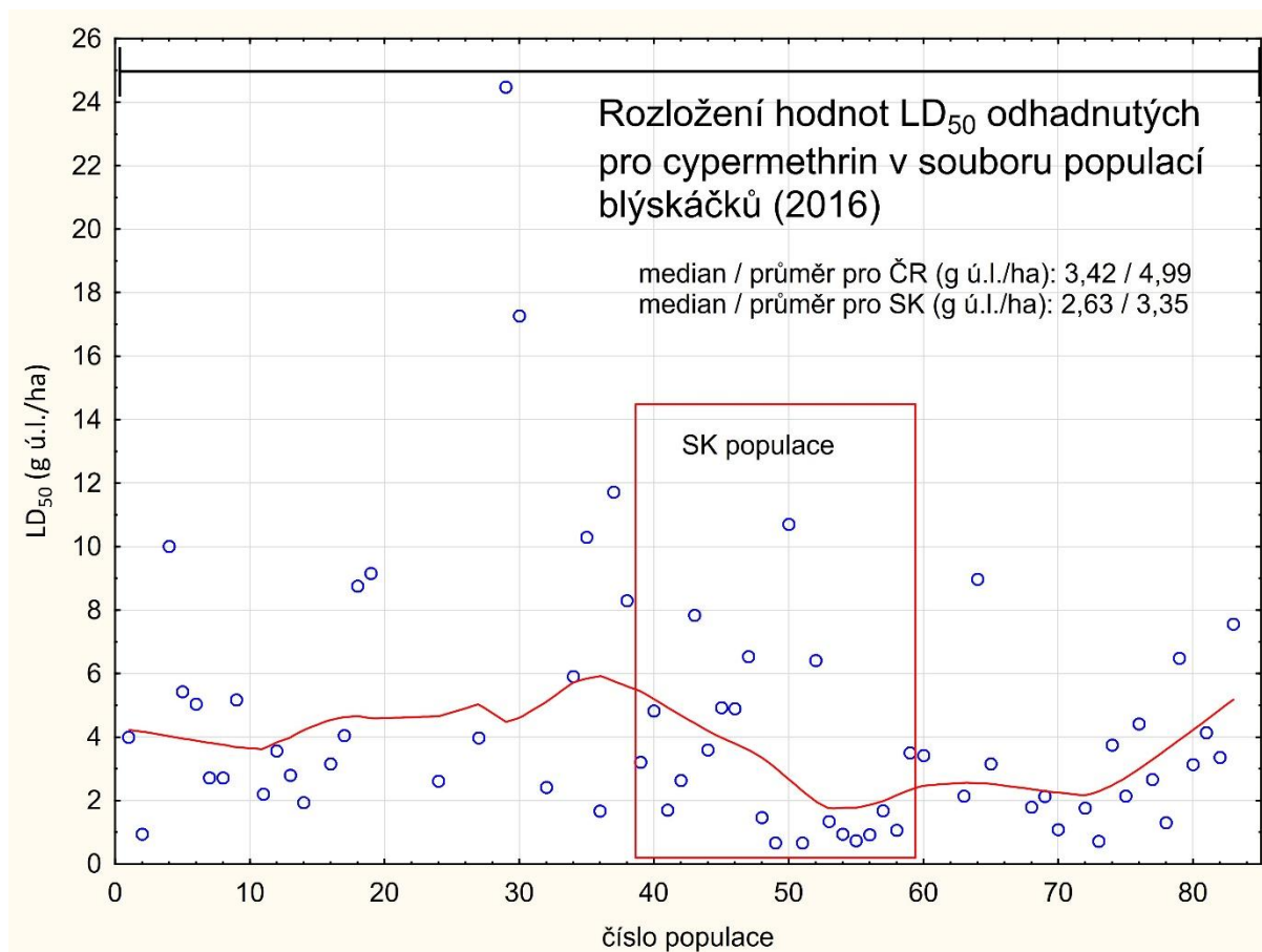
Graf 4 - Rozložení hodnot LD_{50} (g ú.l./ha) odhadnutých pro cypermethrin (probitová regrese) pro testované populace blýskáčků v roce 2016 (každé modré kolečko je jedna testovaná populace). Černá čára vymezuje registrovanou dávku pro cypermethrin v řepce ozimé v ČR (25 g ú.l./ha). Slovenské populace se v grafu nachází v červeném obdélníku. Použitá metoda testování: Adult vial test IRAC 011 version 3 (2016, 66 populací otestováno celkem; 45 z ČR + 21 z SK).
