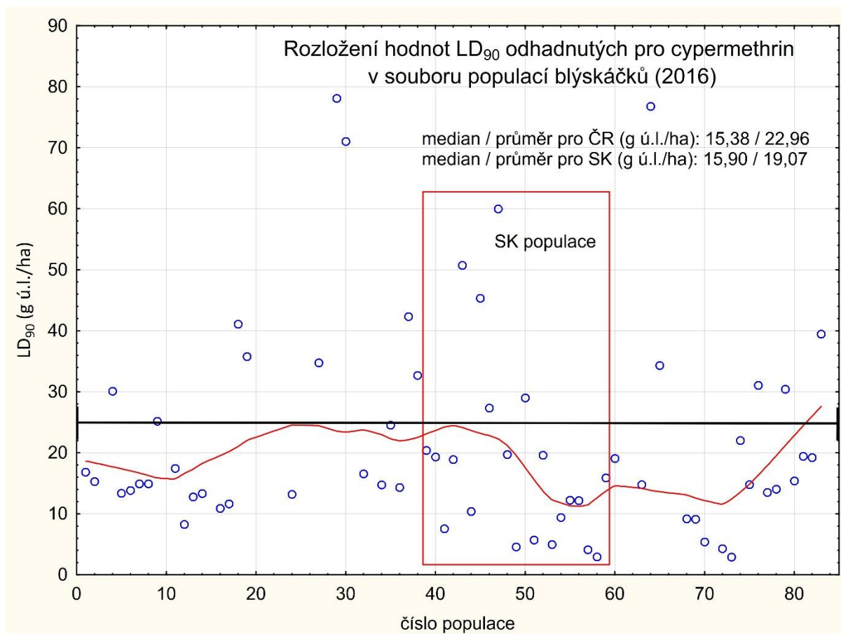
Graf 5 - Rozložení hodnot LD_{90} (g ú.l./ha) odhadnutých pro cypermethrin (probitová regrese) pro testované populace blýskáčků v roce 2016 (každé modré kolečko je jedna testovaná populace). Černá čára vymezuje registrovanou dávku pro cypermethrin v řepce ozimé v ČR (25 g ú.l./ha). Slovenské populace se v grafu nachází v červeném obdélníku. Použitá metoda testování: Adult vial test IRAC 011 version 3 (2016, 66 populací otestováno celkem; 45 z ČR + 21 z SK).
