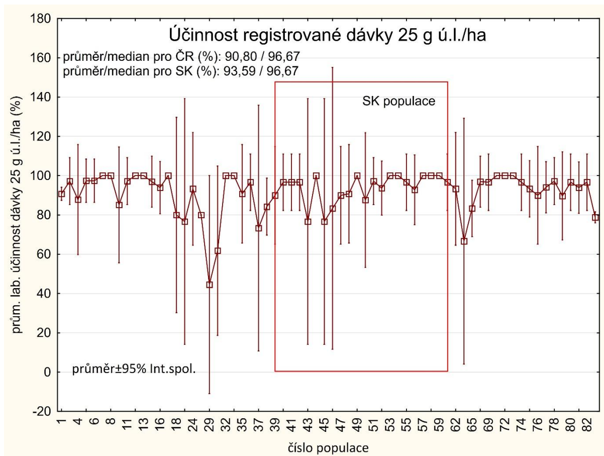
Graf 1 - Hodnoty laboratorních účinností dosažené u jednotlivých populací blýskáčků registrovanou dávkou cypermethrinu v ČR (25 g. ú.l./ha). Čísla populací uvedených v grafu (osa x) odpovídají číslům populací v tabulkách 4a,b a 5a,b. Použitá metoda testování: Adult vial test IRAC 011 version 3 (2016, 66 populací otestováno celkem; 45 populací z ČR, 21 populací z SK).
