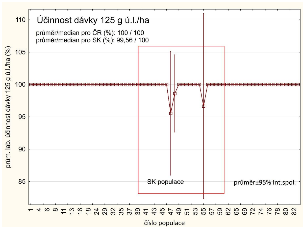
Graf 3 - Hodnoty laboratorních účinností dosažené u jednotlivých populací blýskáčků pětinasobkem dávky registrované (to je 125 g. ú.l./ha). Čísla populací uvedených v grafu (osa x) odpovídají číslům populací v tabulkách 4a,b a 5a,b. Použitá metoda testování: Adult vial test IRAC 011 version 3 (2016, 66 populací otestováno celkem; 45 populací z ČR, 21 populací z SK).
